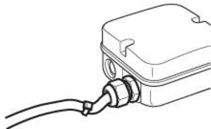
Fig. 1: Ventilatore montato in orizzontale, posa del cavo a U per evitare l'infiltrazione d'acqua.
