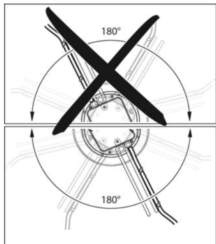
Fig. 2: Posa dei cavi nei ventilatori verticali. I cavi devono avere sempre una disposizione discendente.
